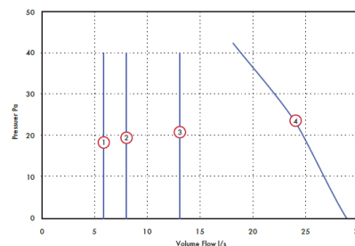
Vent-Axia Response légszállítás tartás
